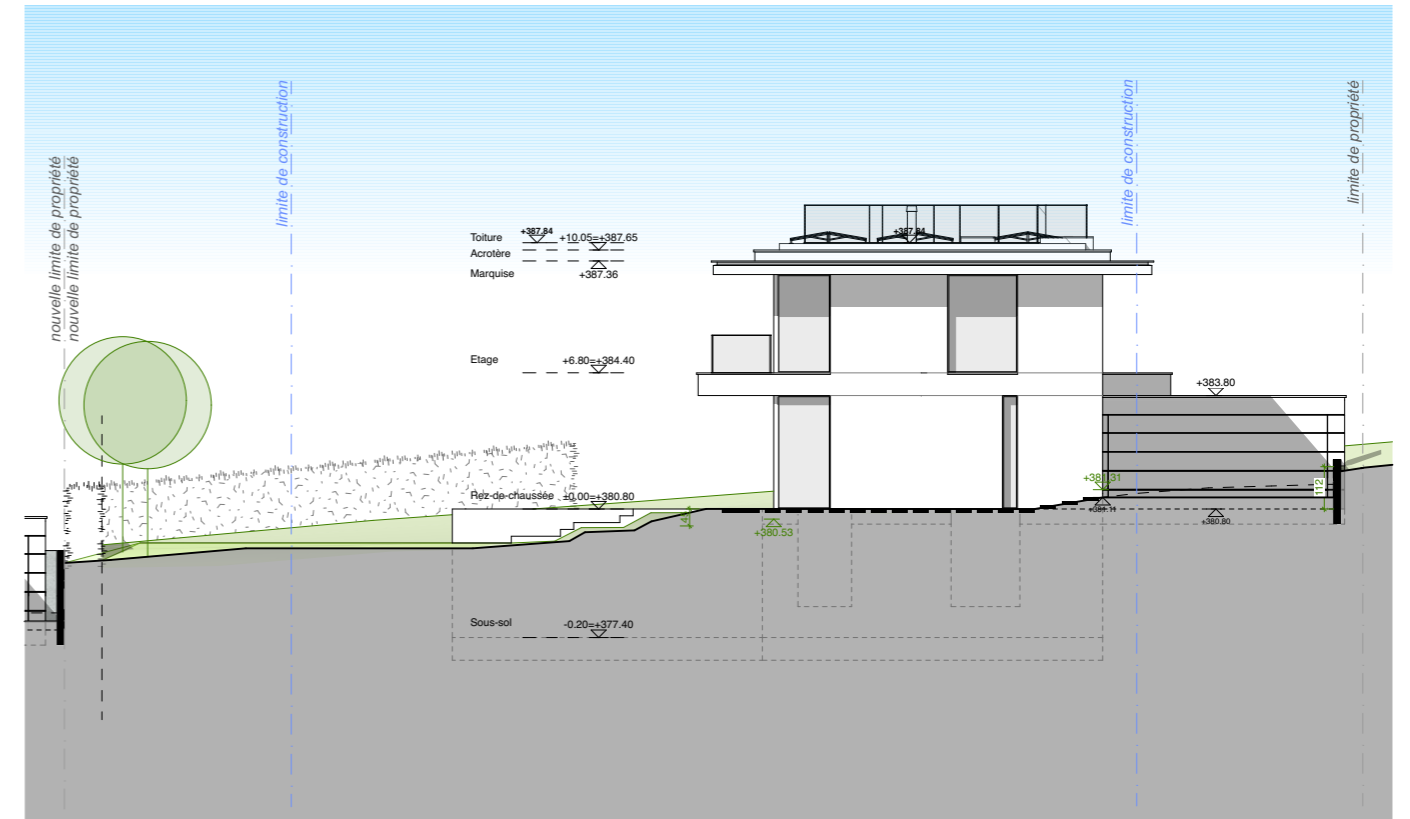
façade nord
