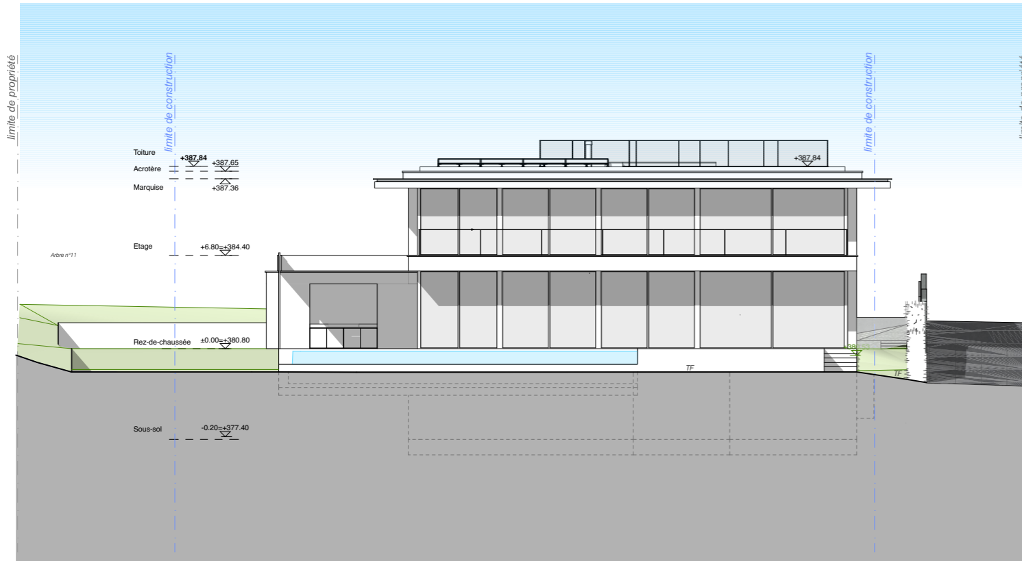
façade est
