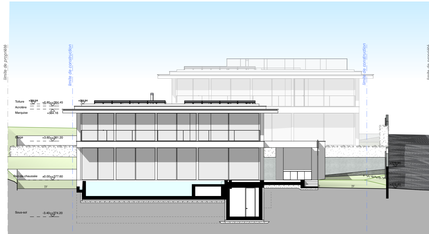
façade est
