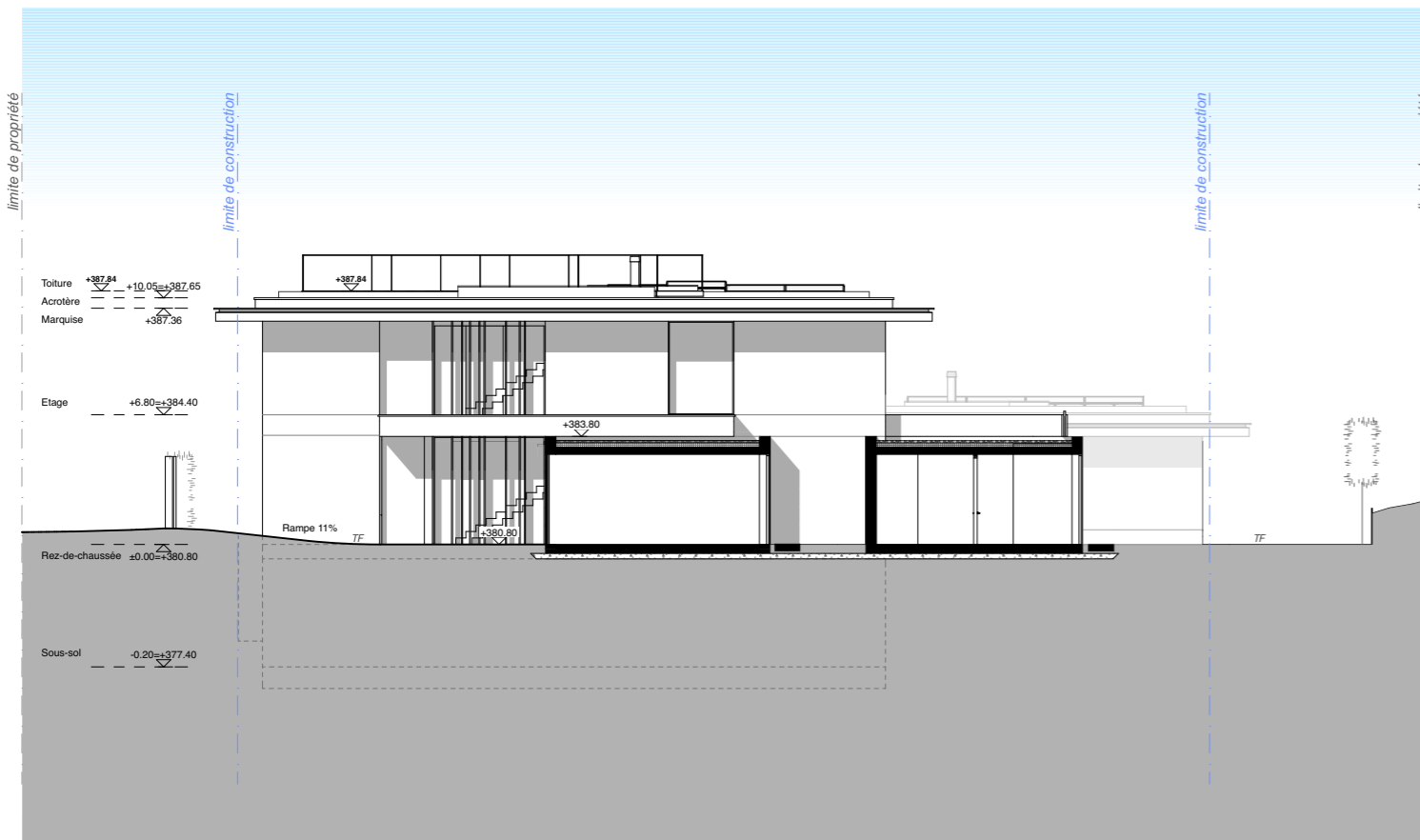
façade nord
