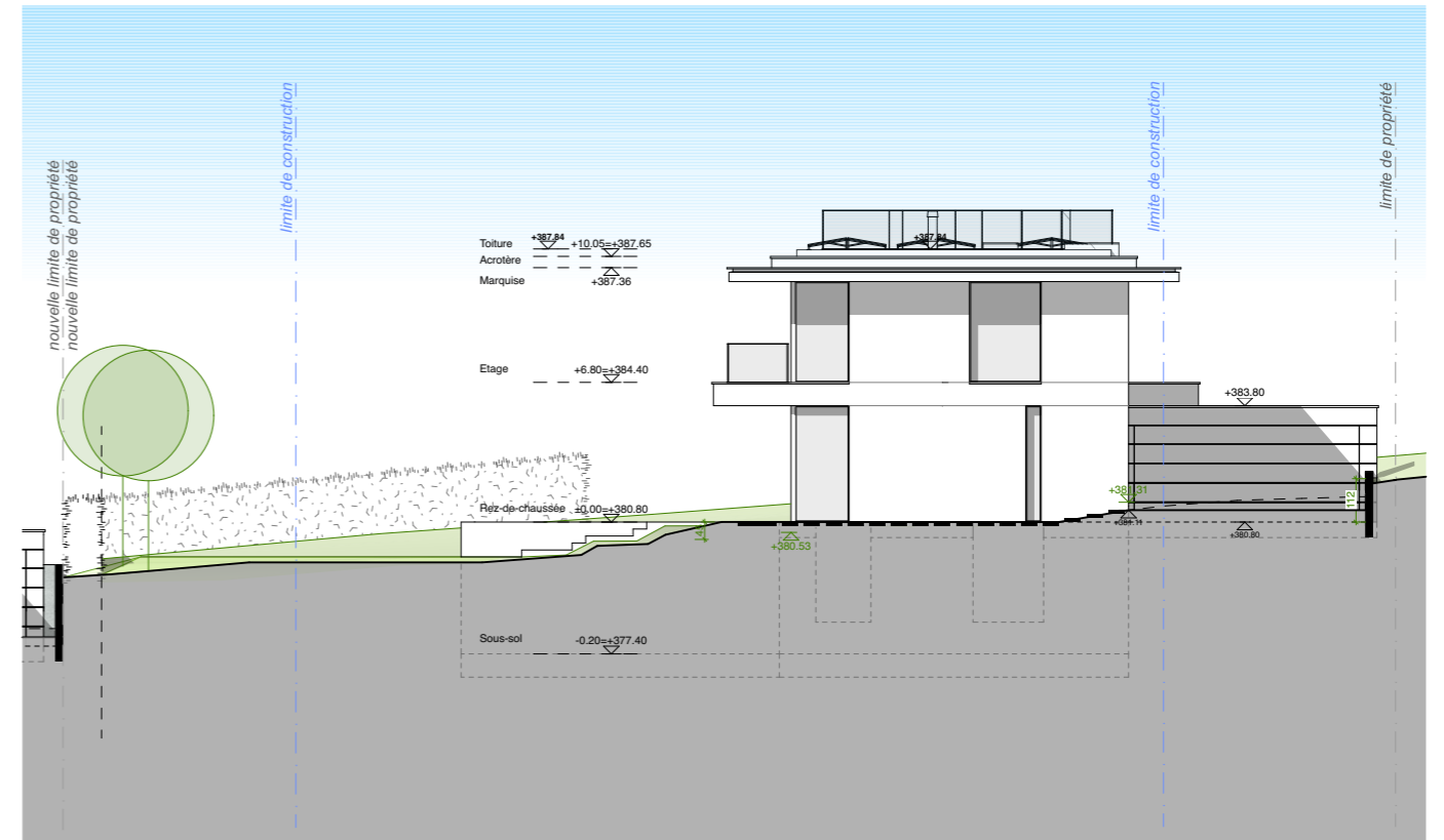
façade nord
